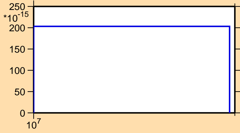
\sigma vs. E for ^{126}\text{Cs} (mt 34)
