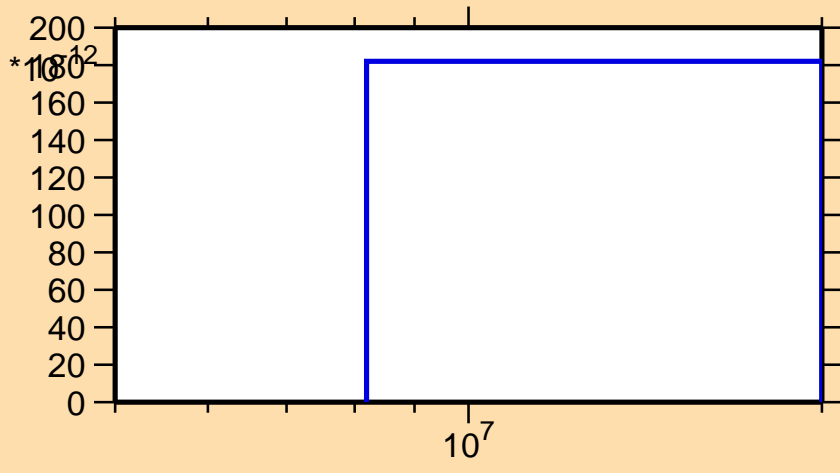
\sigma vs. E for ^{126}\text{Cs} (mt 45)
