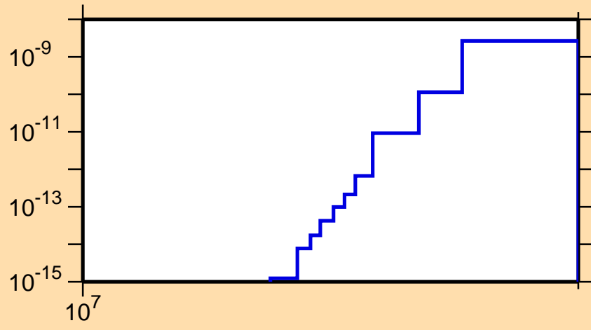
\sigma vs. E for ^{147}\text{Dy}(\text{mt } 34)
