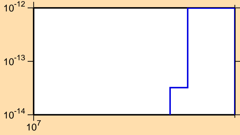
\sigma vs. E for ^{241}\text{Es} (mt 34)
