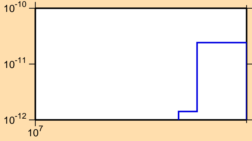
\sigma vs. E for ^{242}\text{Es} (mt 34)
