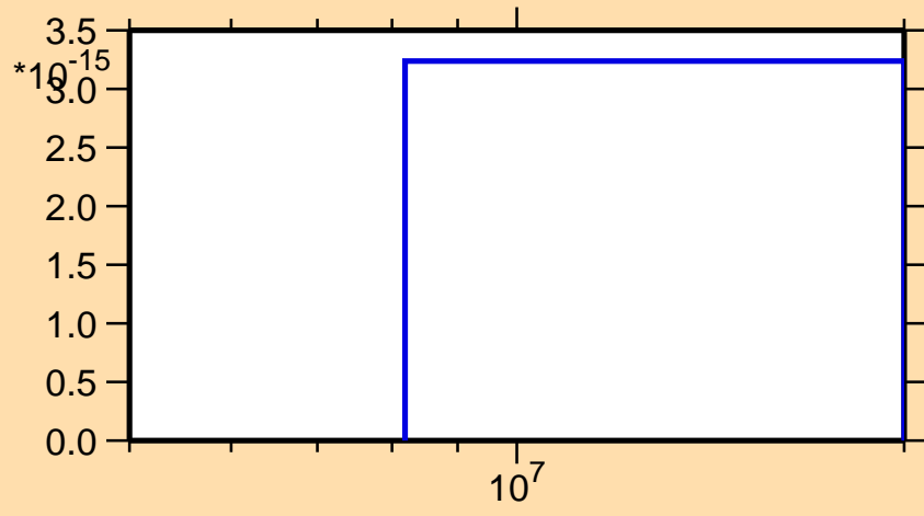
\sigma vs. E for ^{248}\text{Es} (mt 34)
