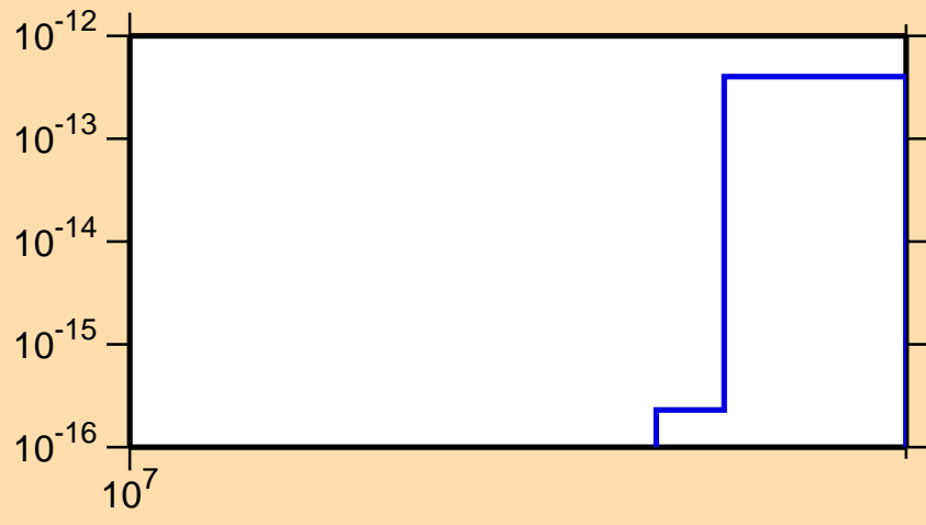
\sigma vs. E for ^{253}\text{Es} (mt 42)
