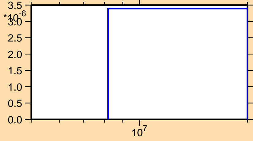
\sigma vs. E for ^{253}\text{Es} (mt 45)
