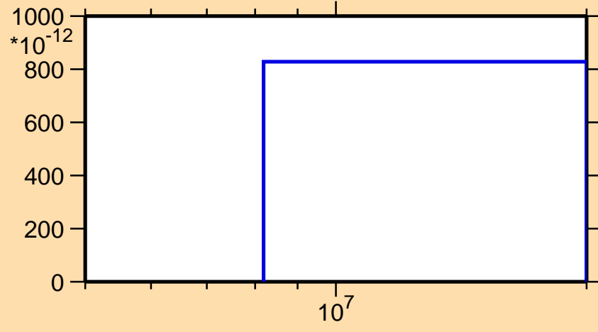
\sigma vs. E for ^{254}\text{Es} (mt 45)
