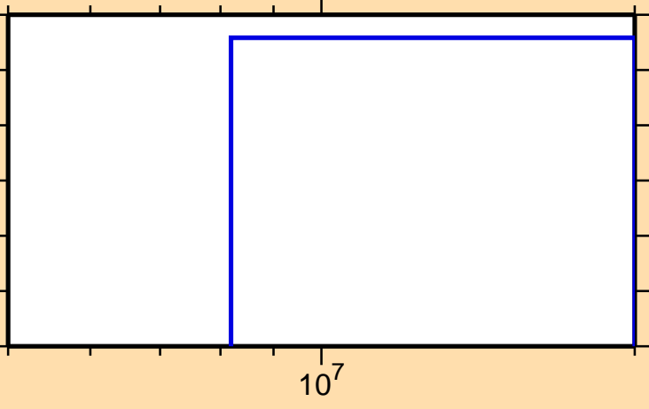
\sigma vs. E for ^{254}\text{Es} (mt 45)
