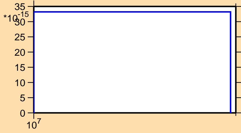
\sigma vs. E for ^{257}\text{Es} (mt 45)
