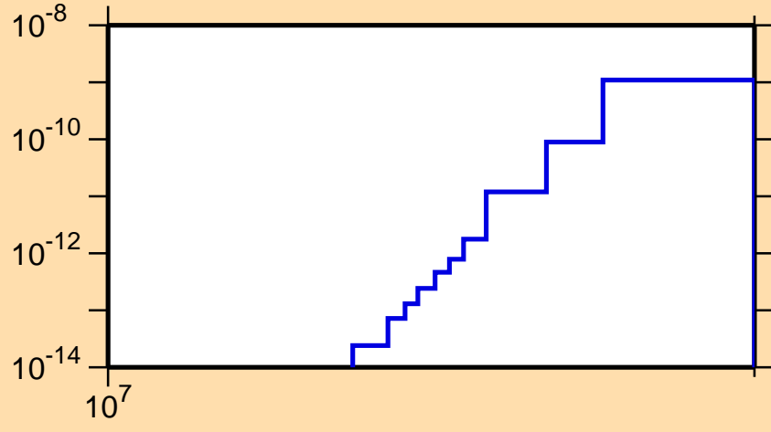
\sigma vs. E for ^{206}\text{Fr}(\text{mt } 34)
