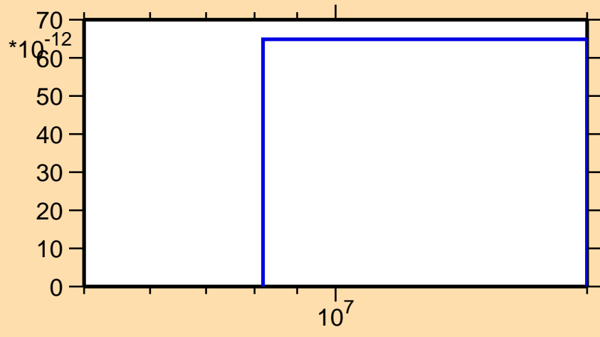
\sigma vs. E for ^{63}\text{Ga}(\text{mt } 34)
