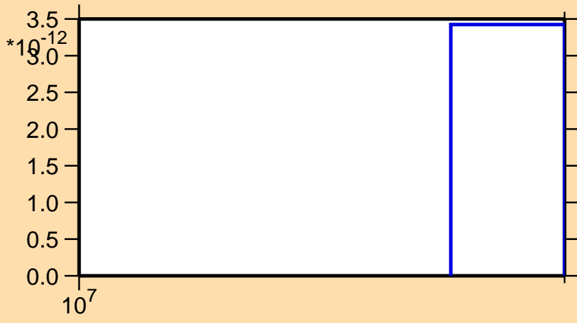
\sigma vs. E for ^{64}\text{Ga}(n,nt)
