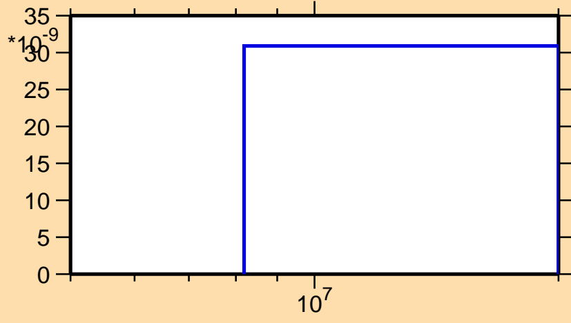
\sigma vs. E for ^{144}\text{Gd}(\text{mt } 45)
