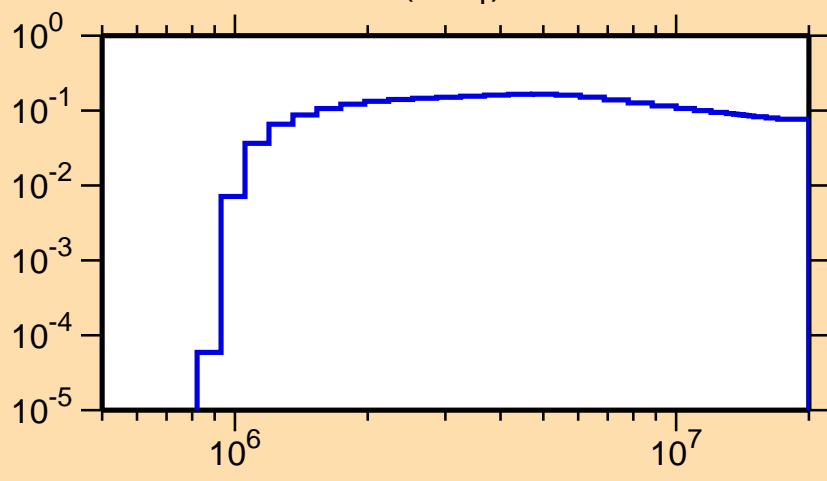
\sigma vs. E for ^{64}\text{Ge}(n,n_1)
