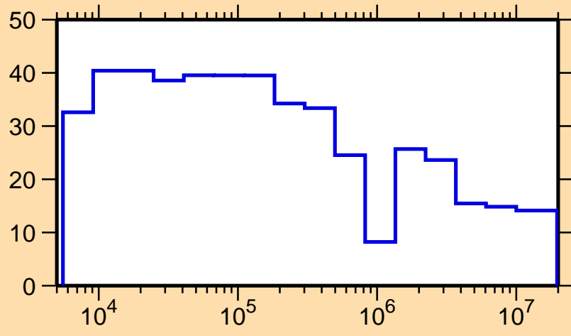
\Delta\sigma/\sigma vs. E for ^{64}\text{Ge}(n,el.)
