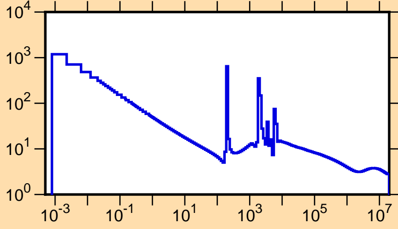
\sigma vs. E for ^{66}\text{Ge}(n,\text{tot.})
