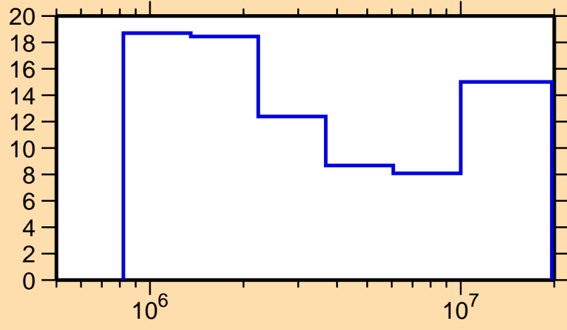
\Delta\sigma/\sigma vs. E for ^{73}\text{Ge}(n,el.)
