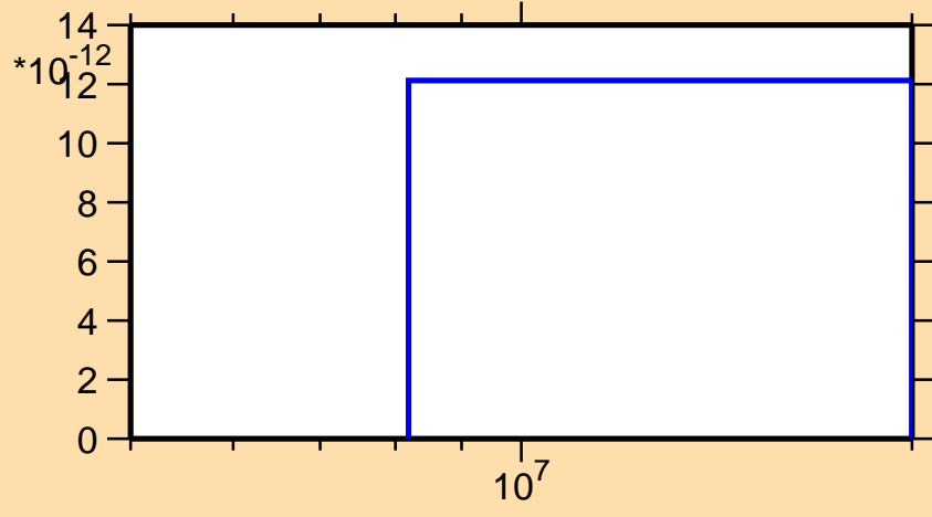
\sigma vs. E for ^{81}\text{Ge}(n,nt)
