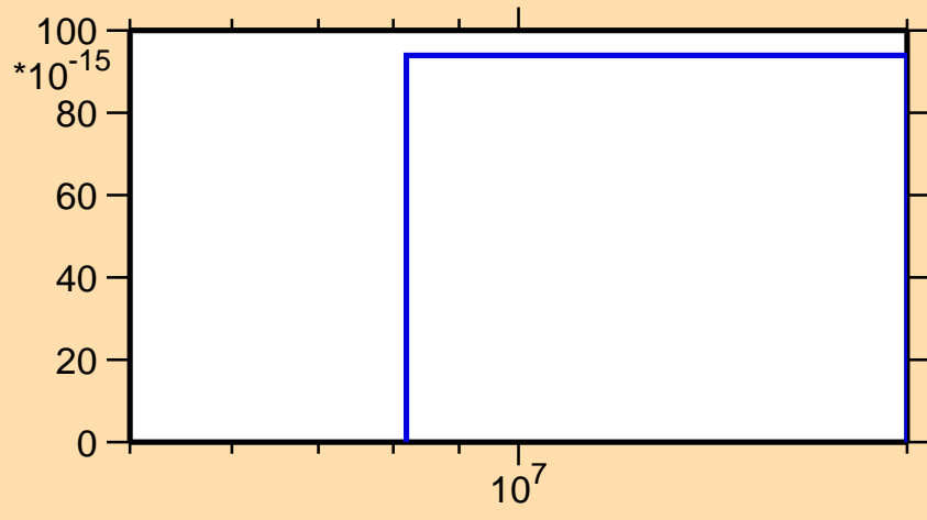
\sigma vs. E for ^{74}\text{Kr}(\text{mt } 34)
