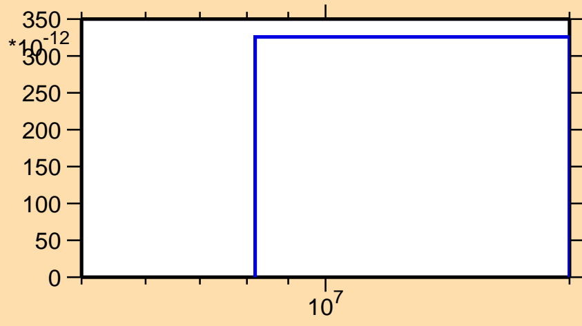
\sigma vs. E for ^{76}\text{Kr}(\text{mt } 45)
