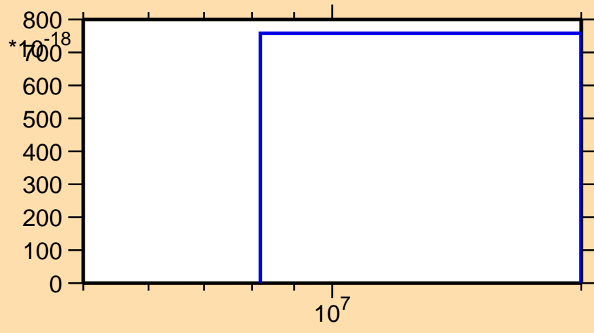
\sigma vs. E for ^{76}\text{Kr}(\text{mt } 34)
