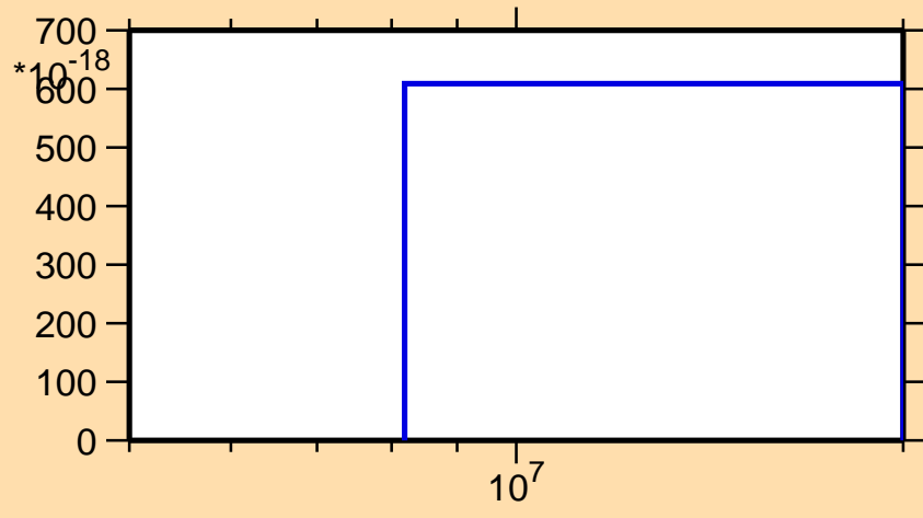
\sigma vs. E for ^{81}\text{Kr}(\text{mt } 34)
