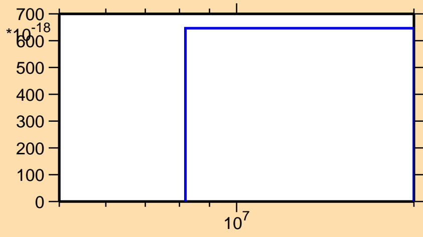
\sigma vs. E for ^{254}\text{Lw}(\text{mt } 42)
