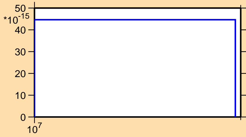
\sigma vs. E for ^{257}\text{Lw} (mt 34)
