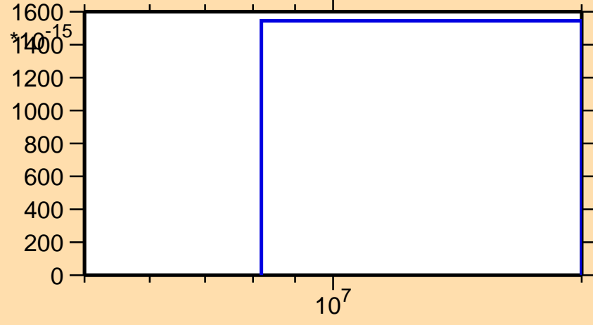
\sigma vs. E for ^{248}\text{Md}(\text{mt } 34)
