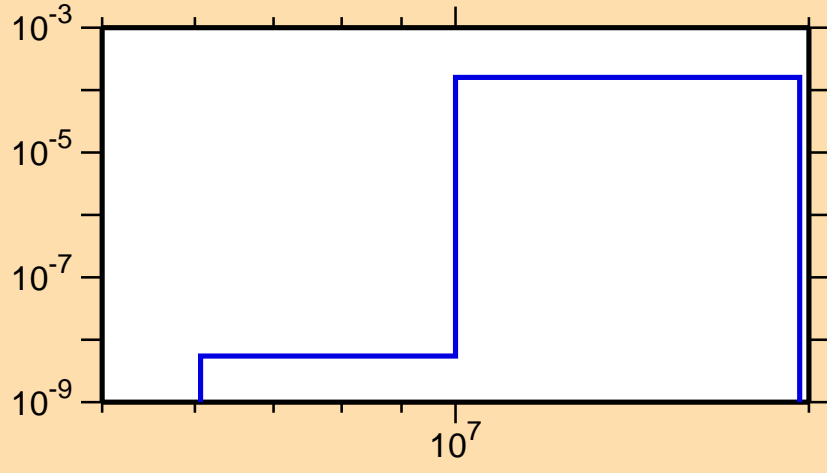
\sigma vs. E for ^{254}\text{Md}(\text{mt } 45)
