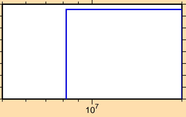
\sigma vs. E for ^{254}\text{Md}(\text{mt } 34)
