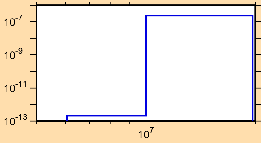
\sigma vs. E for ^{257}\text{Md}(\text{mt } 45)
