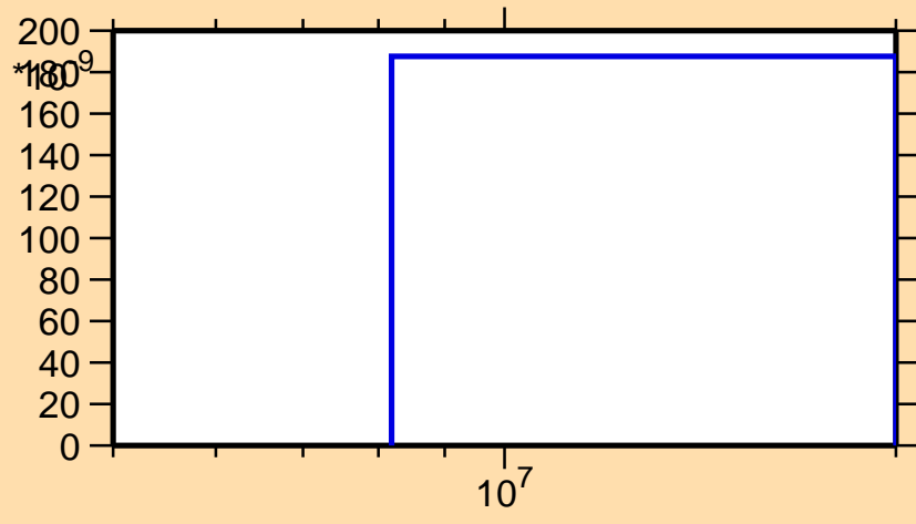
\sigma vs. E for ^{257}\text{Md}(\text{mt } 45)
