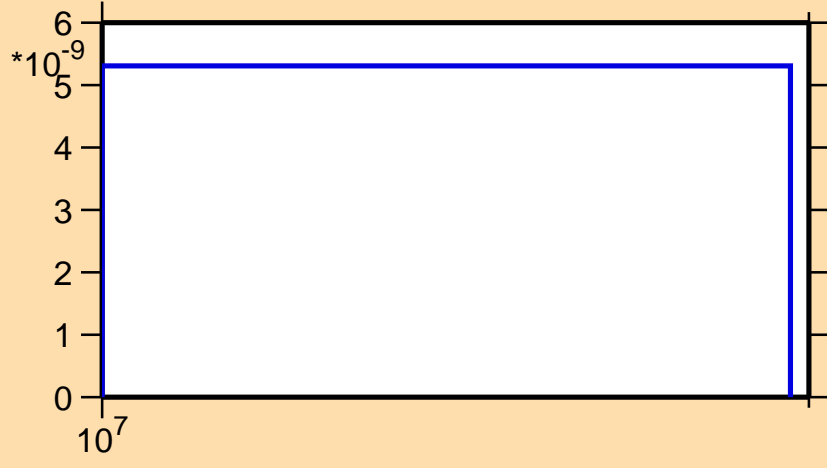
\sigma vs. E for ^{86}\text{Mo} (mt 45)
