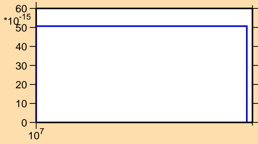
\sigma vs. E for ^{86}\text{Mo} (mt 34)
