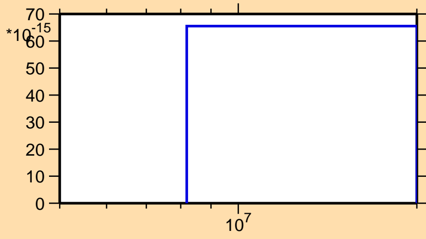
\sigma vs. E for ^{86}\text{Mo}(\text{mt } 34)
