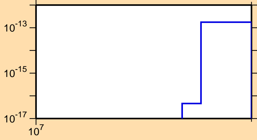
\sigma vs. E for ^{88}\text{Mo} (mt 34)
