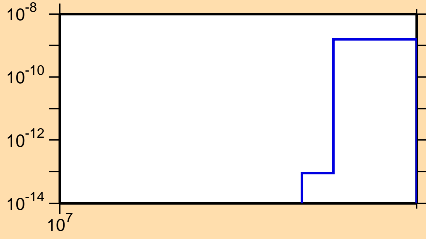
\sigma vs. E for ^{89}\text{Mo} (mt 45)
