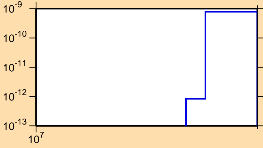
\sigma vs. E for ^{89}\text{Mo} (mt 34)
