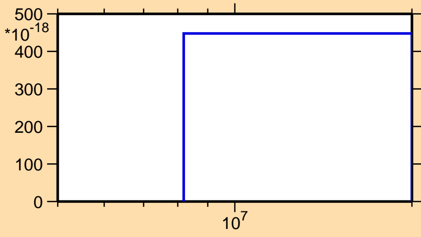
\sigma vs. E for ^{96}\text{Mo}(\text{mt } 45)
