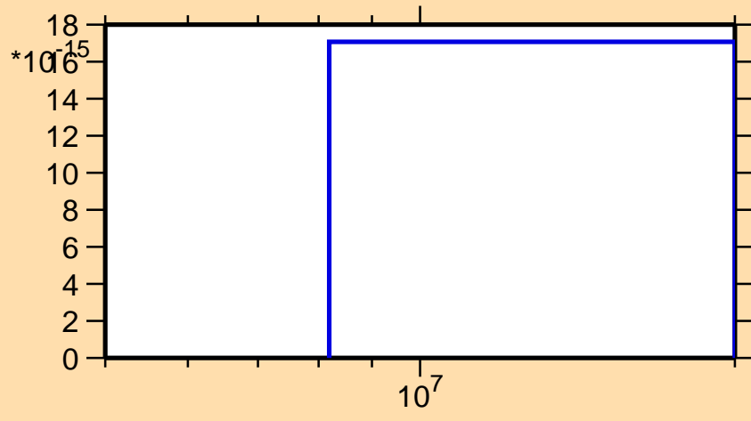
\sigma vs. E for ^{254}\text{No}(\text{mt } 34)
