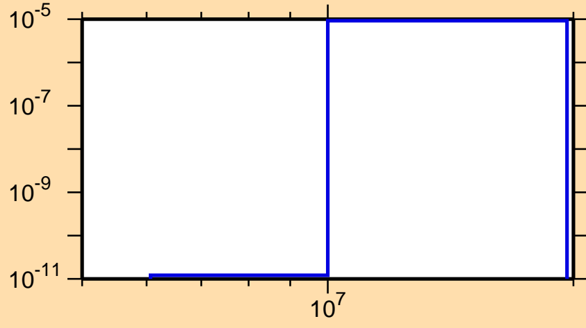
\sigma vs. E for ^{173}\text{Os} (mt 45)
