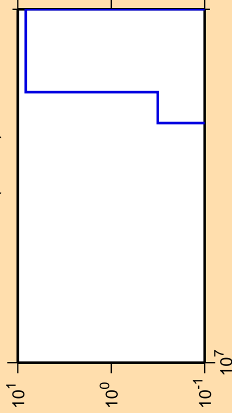
\Delta\sigma/\sigma vs. E for ^{186}\text{Os} (mt 45)
