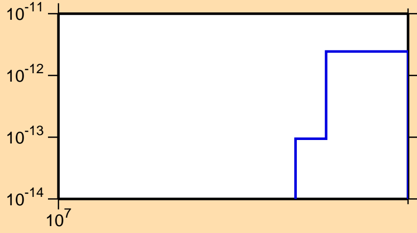
\sigma vs. E for ^{186}\text{Os} (mt 45)
