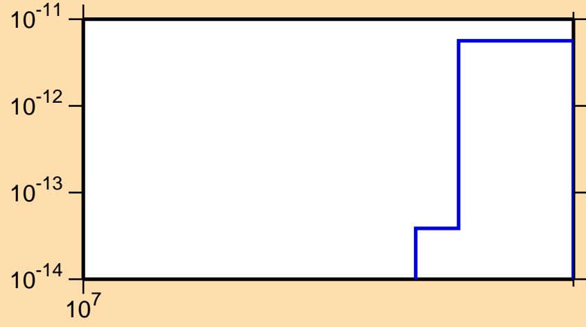
\sigma vs. E for ^{202}\text{Po}(\text{mt } 34)
