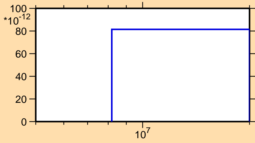
\sigma vs. E for ^{202}\text{Po}(\text{mt } 45)
