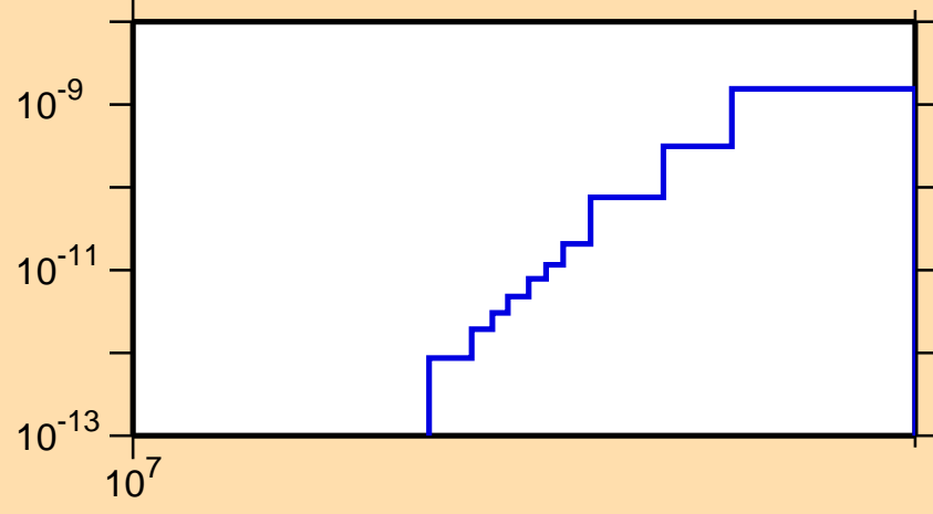
\sigma vs. E for ^{203}\text{Po}(\text{mt } 45)
