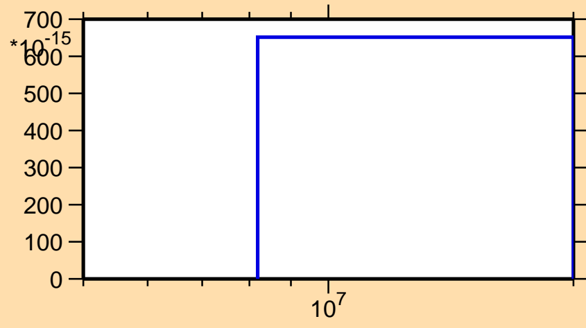
\sigma vs. E for ^{203}\text{Po}(\text{mt } 34)
