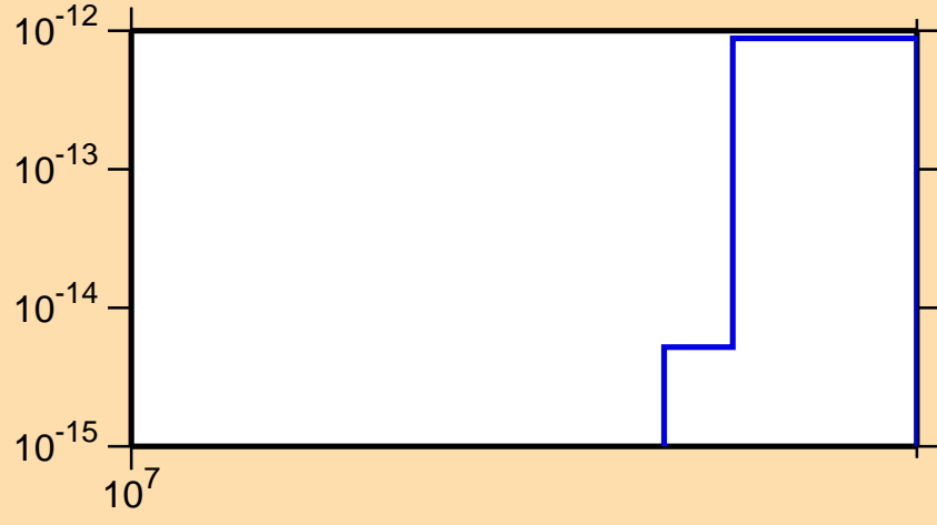
\sigma vs. E for ^{204}\text{Po}(\text{mt } 34)
