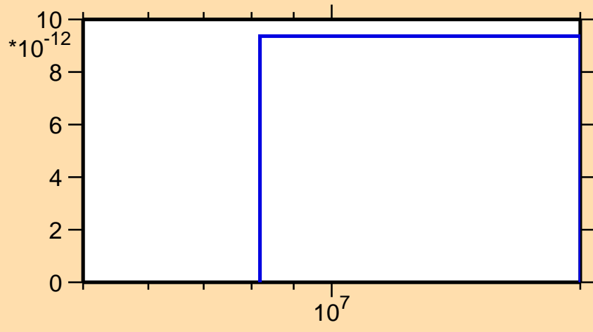
\sigma vs. E for ^{204}\text{Po}(\text{mt } 45)
