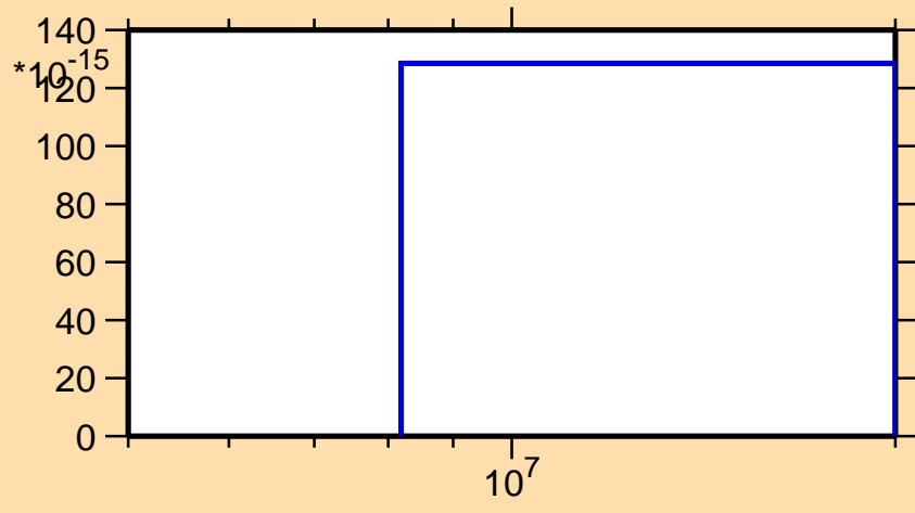
\sigma vs. E for ^{206}\text{Rn}(\text{mt } 34)
