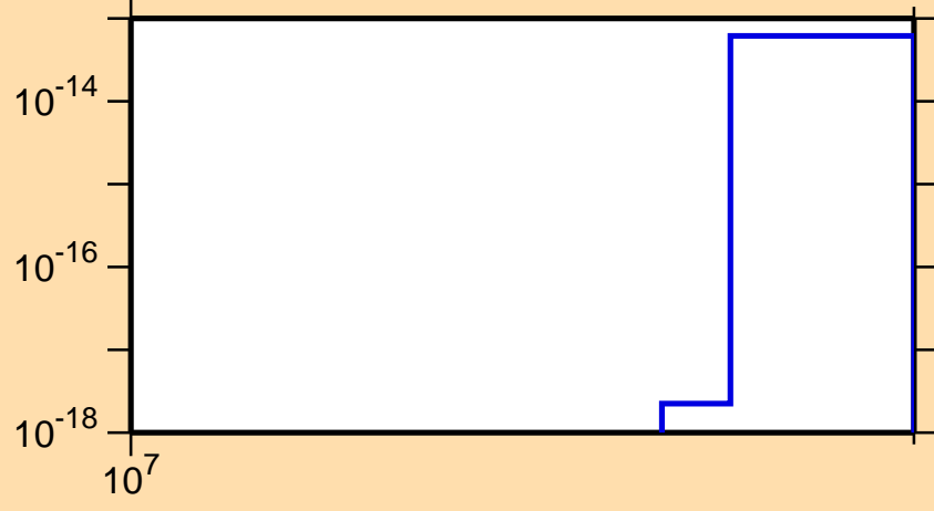
\sigma vs. E for ^{113}\text{Sn}(\text{mt } 45)
