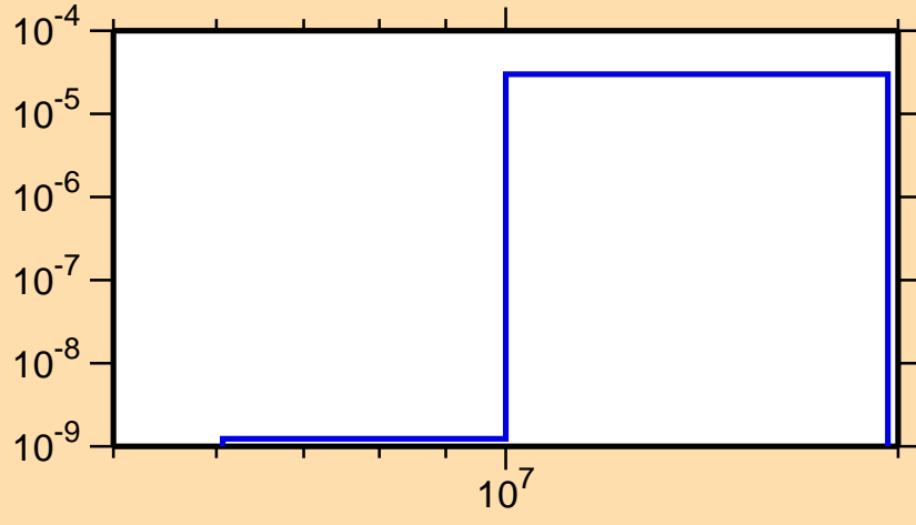
\sigma vs. E for ^{166}\text{Ta}(\text{mt } 45)
