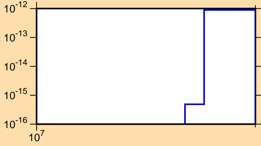
\sigma vs. E for ^{126}\text{Xe}(\text{mt } 45)
