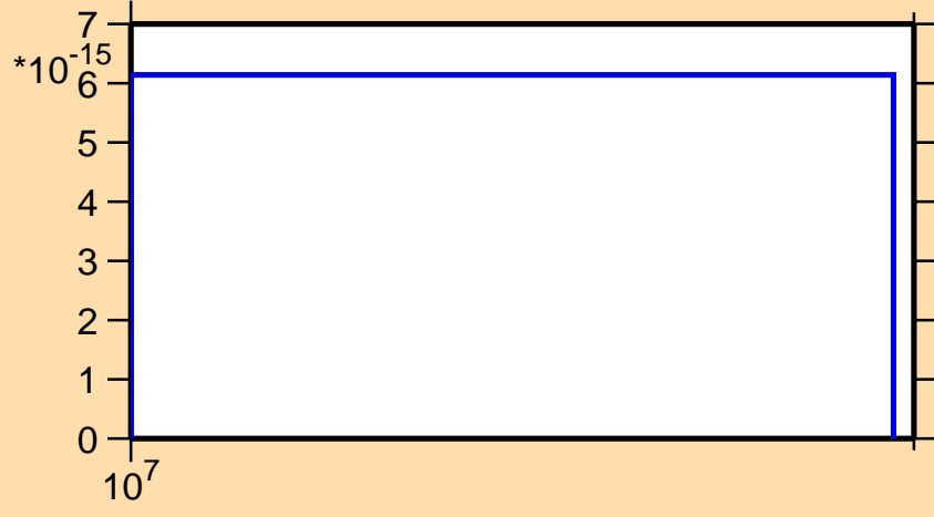
\sigma vs. E for ^{126}\text{Xe}(\text{mt } 45)
