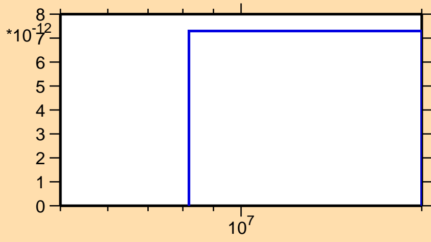
\sigma vs. E for ^{64}\text{Zn}(\text{mt } 45)
